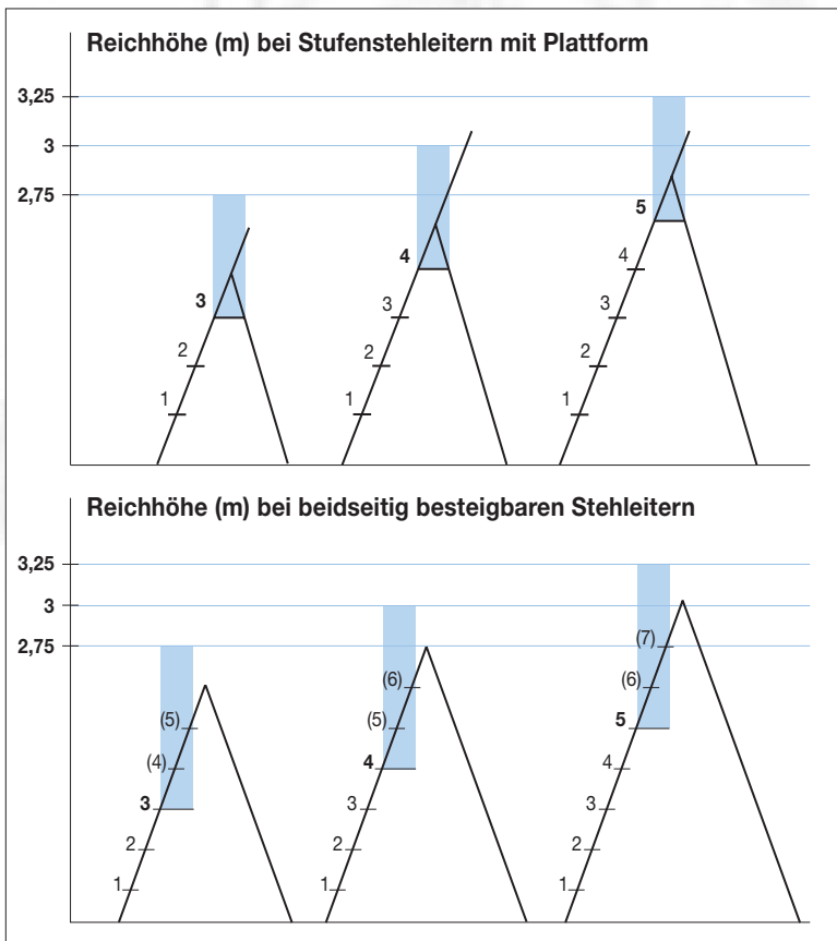
Bild 39: Reichhöhen
